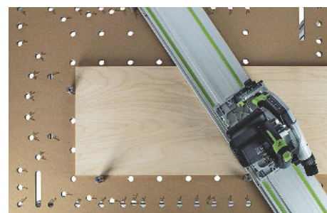
/ Das Lochraster ( \varnothing 20 mm) ist auf genaue Winkelschnitte von 0 bis 100° ausgelegt.
